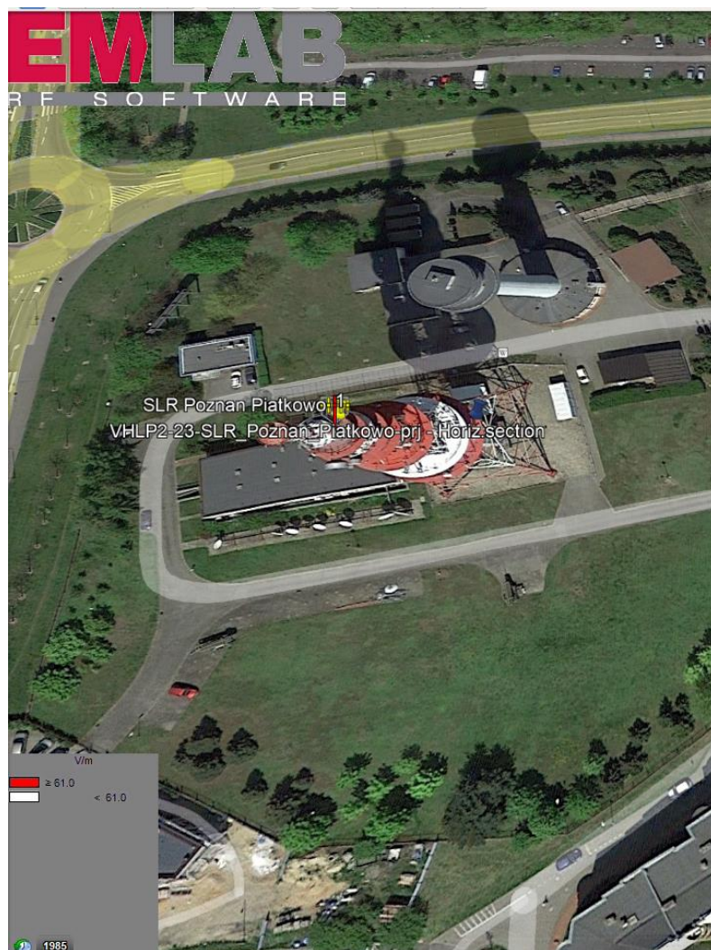
Rys. 2. Rzut poziomy rozkładu pola elektromagnetycznego anteny nowo projektowanej linii radiowej w otoczeniu SLR Poznań Piątkowo przewidzianej do zainstalowania na wysokości 84 m nad poziomem terenu.
