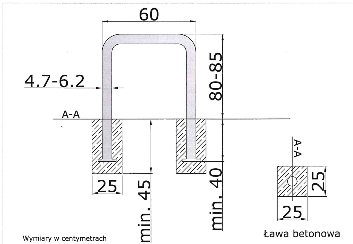
Rys. 25B. Przykładowy stojak rowerowy „odwrócone U” o innych dopuszczalnych wymiarach.
