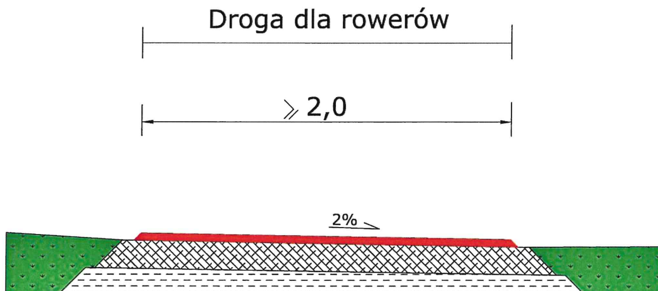
Rys. 12C. Konstrukcja drogi dla rowerów bez obrzeży (krawężników).
