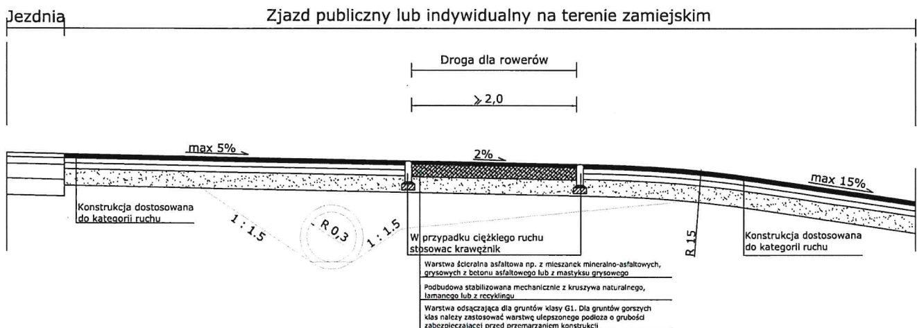
Rys. 12E. Przykład konstrukcji drogi dla rowerów na przecięciu zjazdu indywidualnego (droga zamiejska). Należy zwrócić uwagę, że sytuacja wysokościowa (spadki poprzeczne) może być zupełnie inna. Patrz też przykład na rys. 12F oraz rys. 13.
