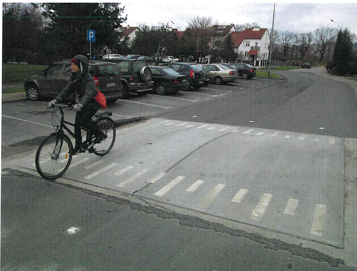
Fot. 1: Prefabrykowany płytowy próg zwalniający, optymalny z punktu widzenia ruchu rowerowego ze względu na obniżenia przy krawędzi jezdni (Wrocław).
