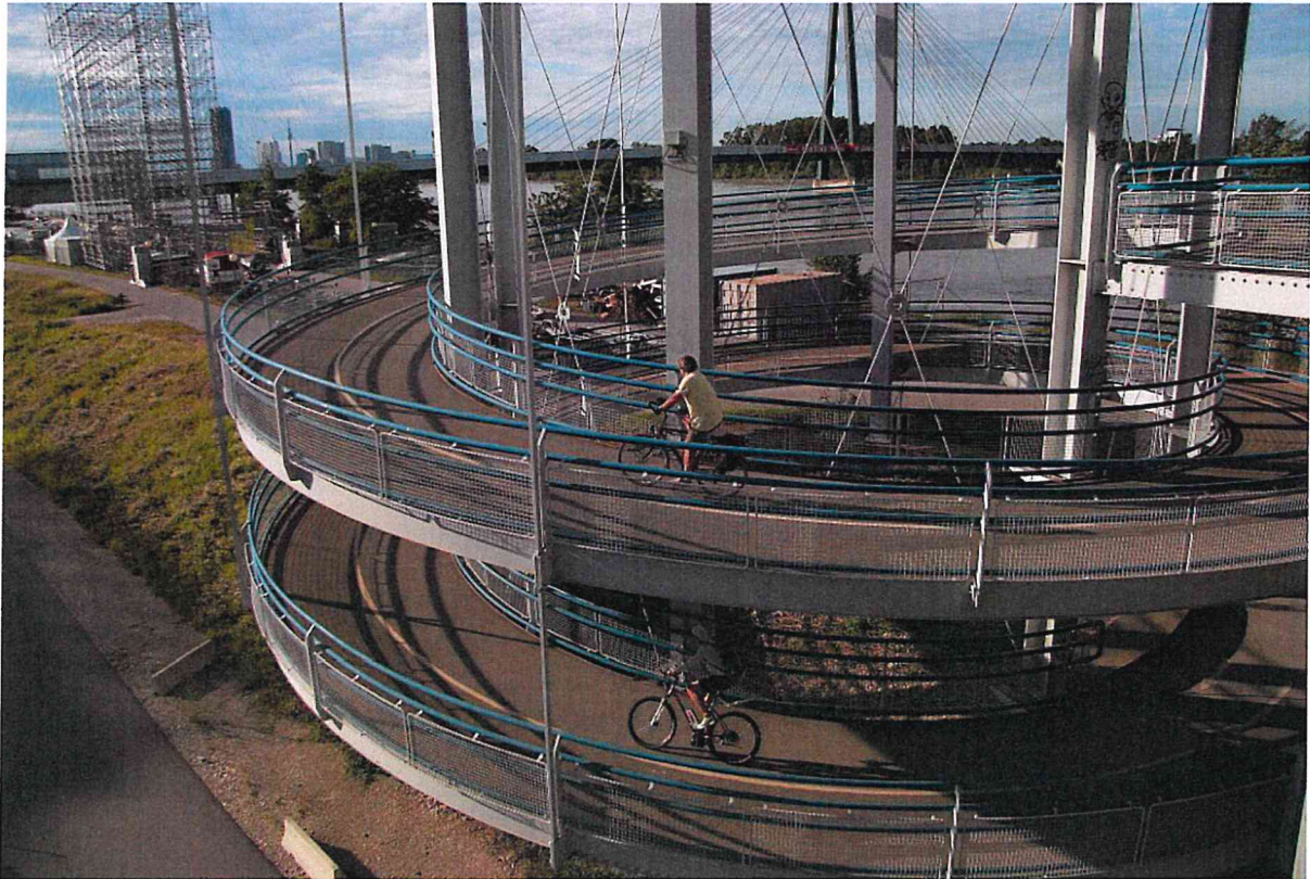
Fot. 15. Pochylnia ślimakowa prowadząca z brzegu Dunaju na drogę dla rowerów zlokalizowaną w dolnym poziomie mostu Praterbrücke. Widoczna prawidłowa orientacja pochylni: w lewo w dół, zapewniająca większy promień łuku rowerzystom jadącym z większą szybkością w dół i minimalizująca ryzyko kolizji. Zwraca uwagę wysoka balustrada z wybaczną poręczą. Wiedeń, Austria.
