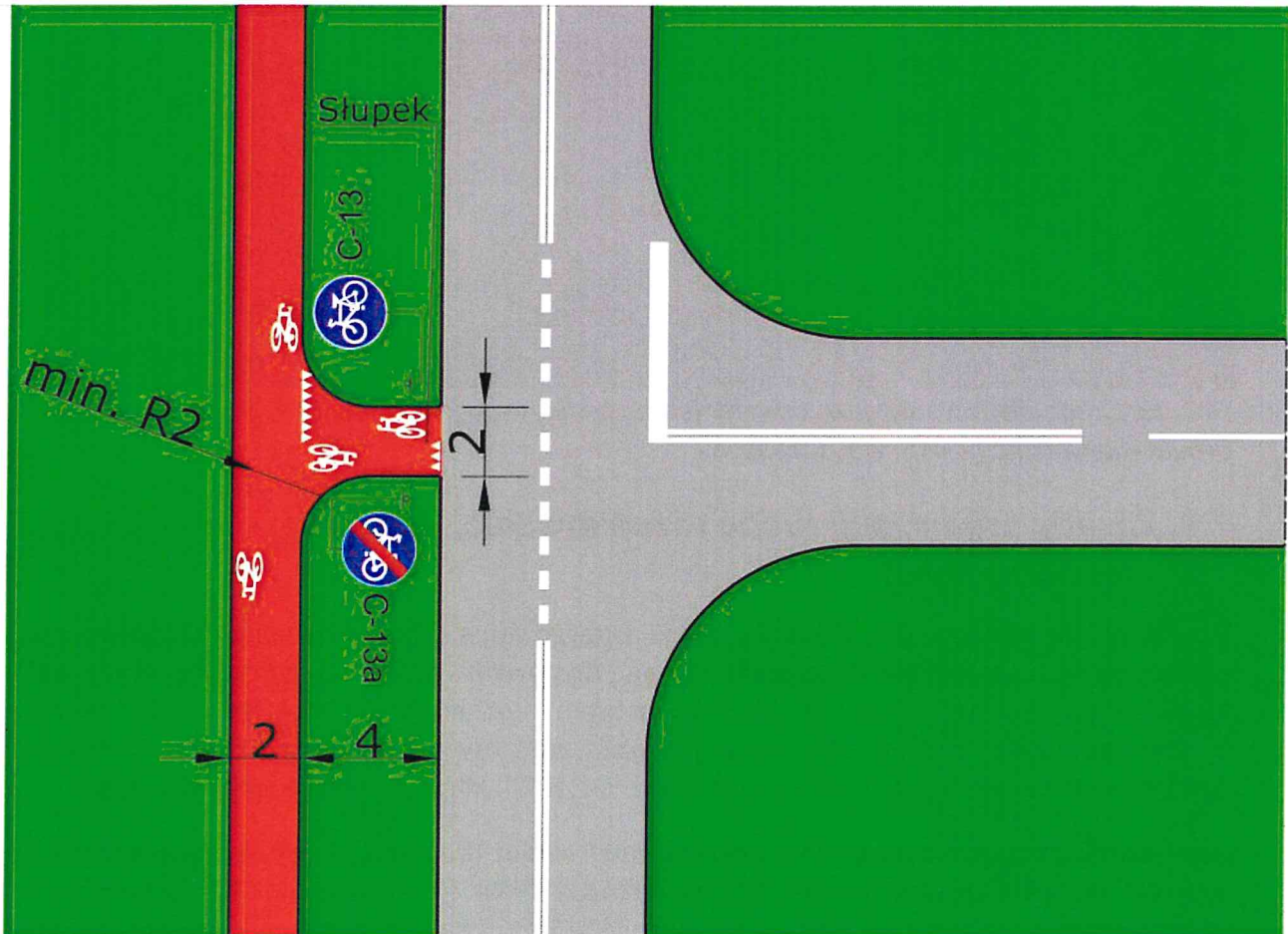
Rys. 23B. Przykład drogi z drogą dla rowerów skomunikowaną na skrzyżowaniu w kształcie litery T („teowym”) przez czwarty wlot. Analogiczne rozwiązania należy stosować w przypadku wszelkich innych źródeł i celów podróży zlokalizowanych po stronie przeciwnej niż biegnie droga dla rowerów. (Część oznakowania pominięto).
