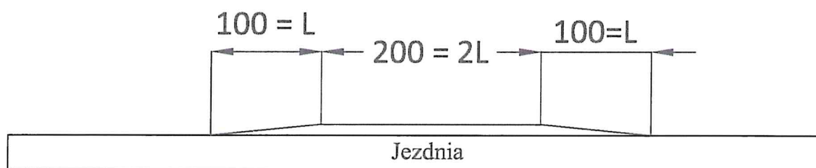
Rys. 1. Płytkowy próg zwalniający – przekrój podłużny
