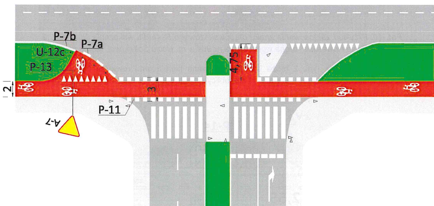
Rys. 20D. Droga dla rowerów i przejazdy dla rowerzystów ze śluzami do skrótu w stronę skrzyżowania (typu 3, pośrodku) i do skrótu na drodze dla rowerów (typu 4, w lewym narożniku) umożliwiającymi bezpieczne pokonanie skrzyżowania na relacjach nie obsługiwanych drogami dla rowerów. Część oznakowania pominięto.
