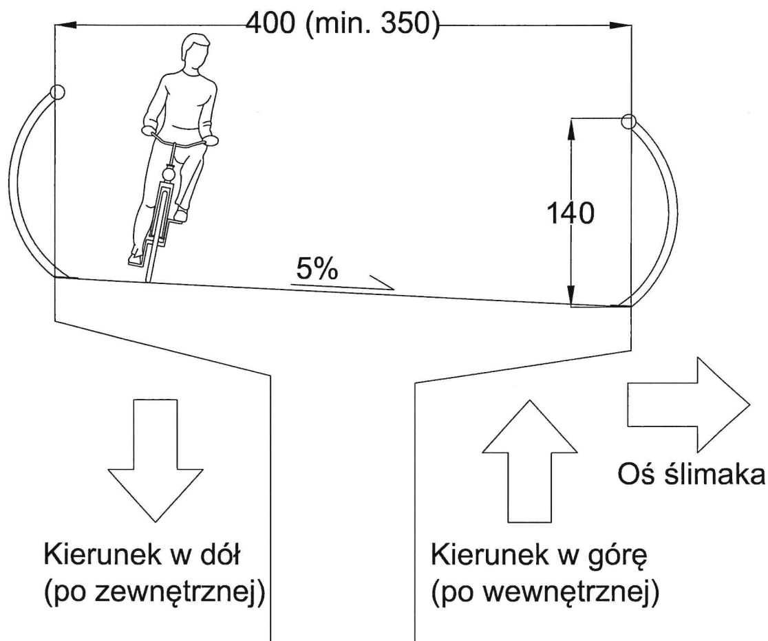
Rys. 24B. Przekrój poprzeczny pochylni ślimakowej. Droga dla rowerów zawsze musi być pochylona w przekroju do wewnątrz w kierunku osi ślimaka. Rowerzysta zjeżdżający w dół zawsze musi znajdować się po zewnętrznej stronie pochylni. Pochylnia (jak i wszystkie obiekty takie jak kładki) powinny być wyposażone w balustrady o przekroju poprzecznym jak na szkicu, aby minimalizować ryzyko zaczepienia o nie kierownicą roweru (w przypadku kolizji z barierą rowerzysta bezpiecznie przyjmuje zderzenie przedramieniem).
