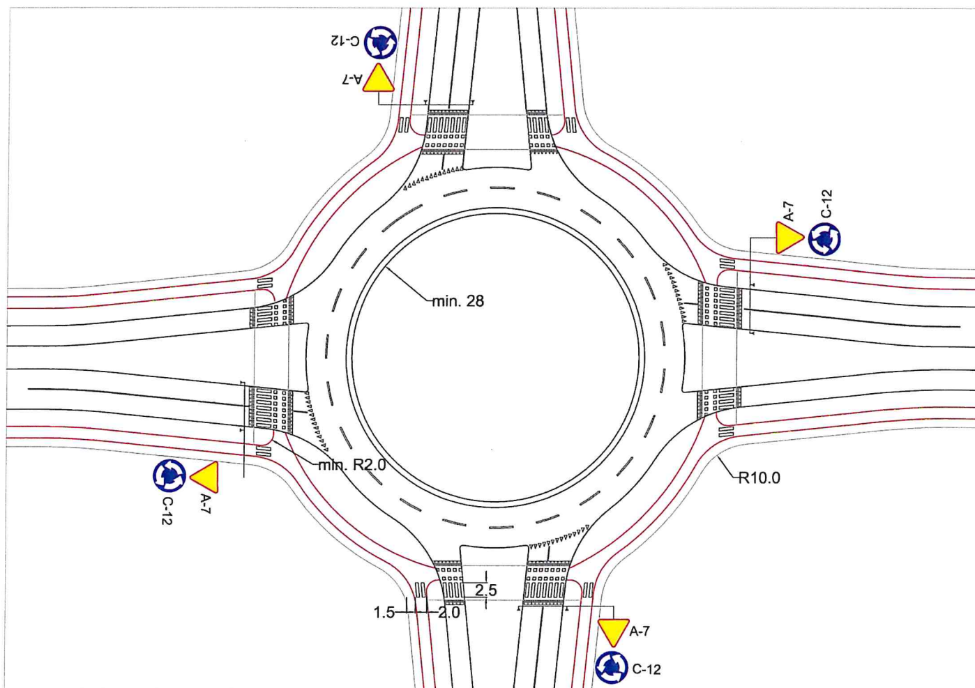
Rys. 22A. Rondo średnie (lub duże) z dwoma pasami ruchu na obwodni i pierwszeństwem rowerzystów na przejazdach dla rowerzystów przez wloty wynikającym z art. 27 ust. 1a ustawy Prawo o Ruchu Drogowym oraz oznakowania. Pierwszeństwo jest podkreślone progami zwalniającymi na wlotach i wylotach ronda. Zwraca uwagę jeden pas ruchu na każdym wylocie ronda: skraca to drogę pieszym i uniemożliwia wyprzedzanie się samochodów opuszczających skrzyżowanie. Część oznakowania (np. znaki pionowe C-13) pominięto dla czytelności rysunku.
