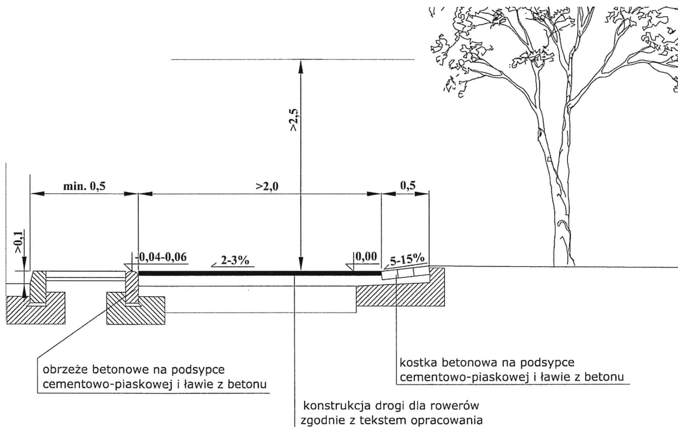
Rys. 12A. Przekrój poprzeczny dwukierunkowej drogi dla rowerów o nawierzchni bitumicznej, zamkniętej obrzeżem i opaską z kostki brukowej oddzielającą ją od chodnika (nie przedstawiony na rysunku).
