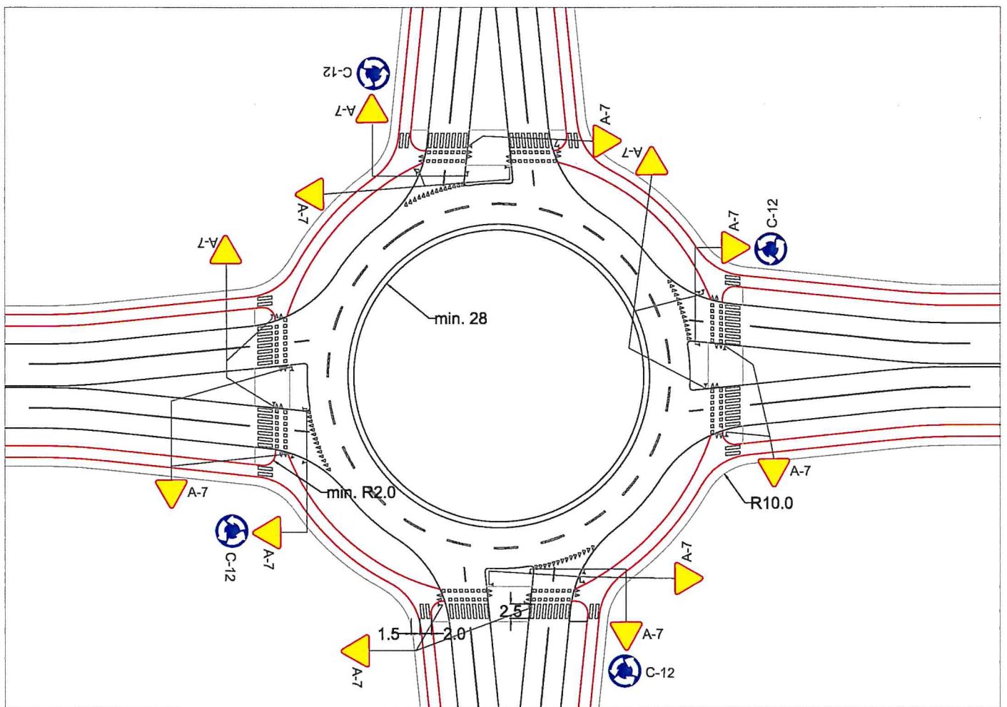
Rys. 22B. Przykład dużego lub średniego ronda z dwoma pasami ruchu na obwiedni i pierwszeństwem na wlotach i przejazdach rowerowych przez wloty ustalonymi znakami drogowymi. Zwraca uwagę umiejscowienie znaków A-7 i C-12 przeznaczonych dla kierujących wjeżdżających na rondo, które znajdują się między przejazdem dla rowerzystów a obwiednią ronda. Znaki A-7 (lub B-20) na drodze dla rowerów mogą być w rozmiarze „mini” i na wysokości 1,0 m nad niweletą drogi dla rowerów. Rozwiązanie stosuje się, kiedy przepis art. 27 ust. 1a nie ma zastosowania (niektóre ronda turbinowe, ronda o bardzo „szybkiej” geometrii wylotów, ronda z łącznicami).
