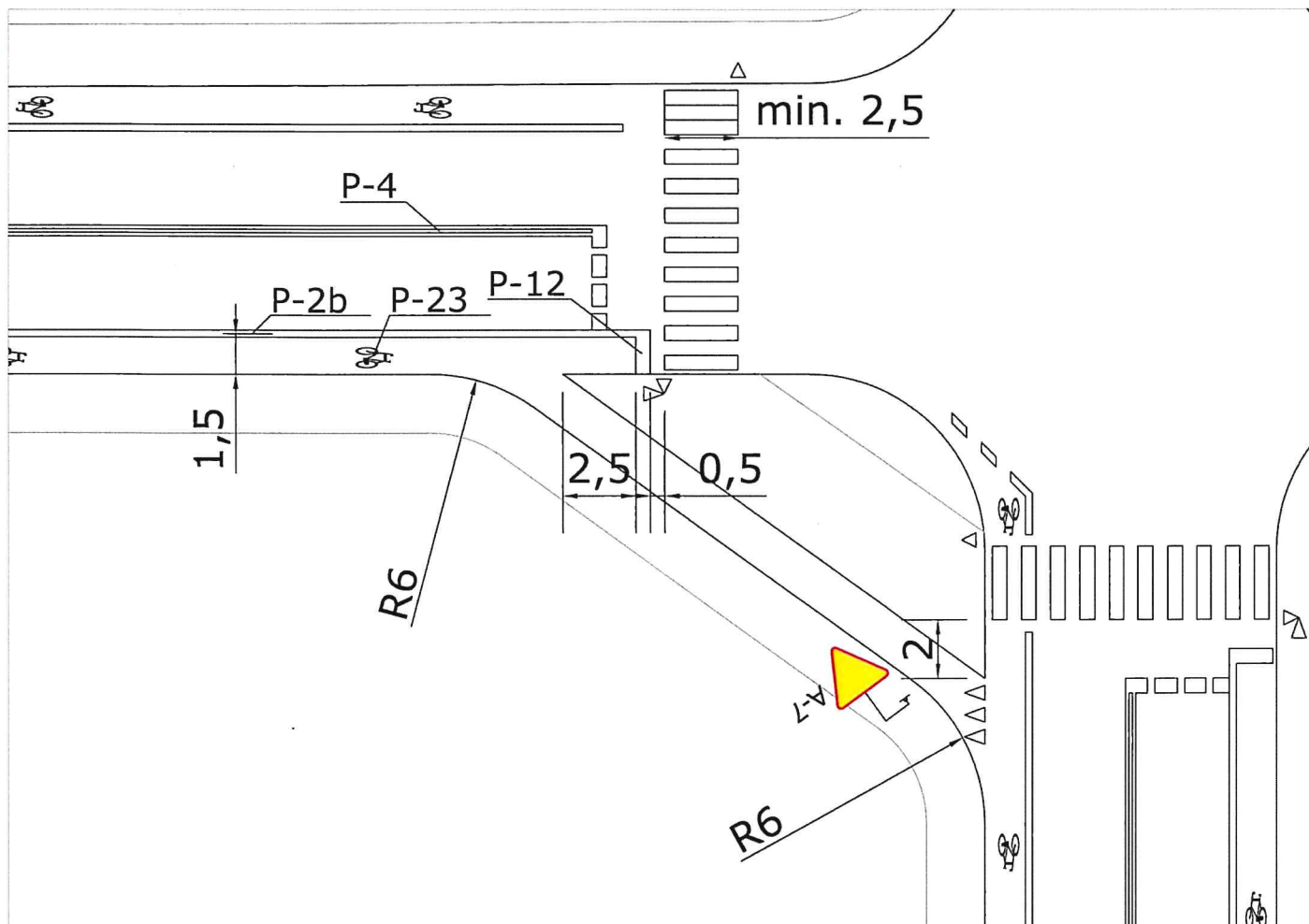
Rys. 20F. Przykład „okrojonej” śluzi typu 1 (linia zatrzymań dla rowerzystów wysunięta o 1,5 m względem linii zatrzymań dla pozostałych pojazdów) wraz z łącznicą umożliwiającą ominięcie skrzyżowania na relacji w prawo i sygnalizatora przed nim. Część oznakowania pionowego pominięto.
