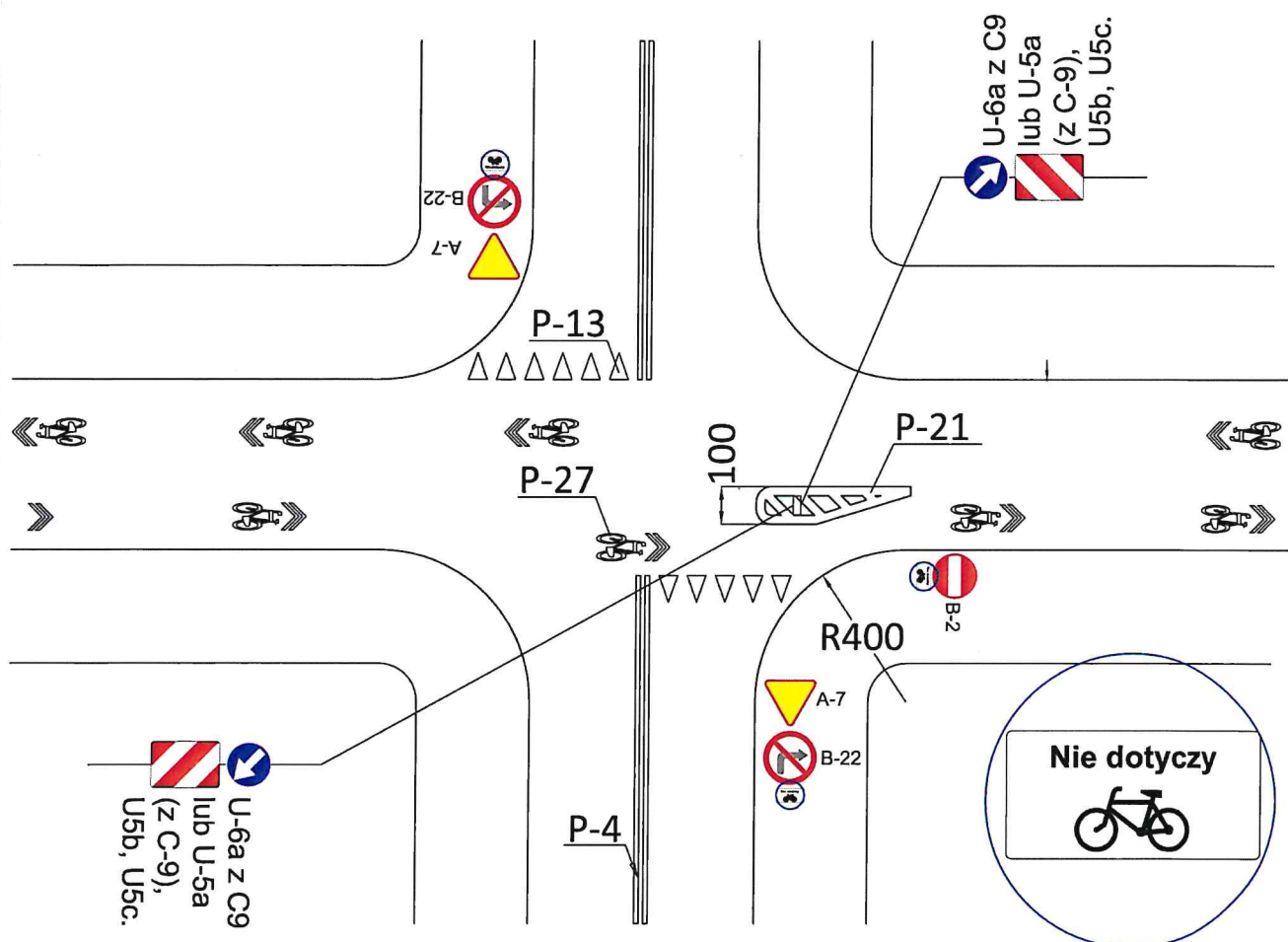
Rys. 4. Przykładowa organizacja dwukierunkowego ruchu rowerowego na jezdni jednokierunkowej – skrzyżowanie z ustalonym pierwszeństwem. Ruch „pod prąd” dopuszczony jest oznakowaniem poziomym P-27, znaki dla kierunku pod prąd umieszcza się zgodnie z opisem w tekście (punkt 4.3). Na wlocie z kontraruchem wyznacza się powierzchnię wyłączoną z ruchu (P-21) rozdzielającą kierunki a na niej umieszcza się słupek przeszkodowy (podatny) lub tablicę kierującą (U-5a lub U-6a).
