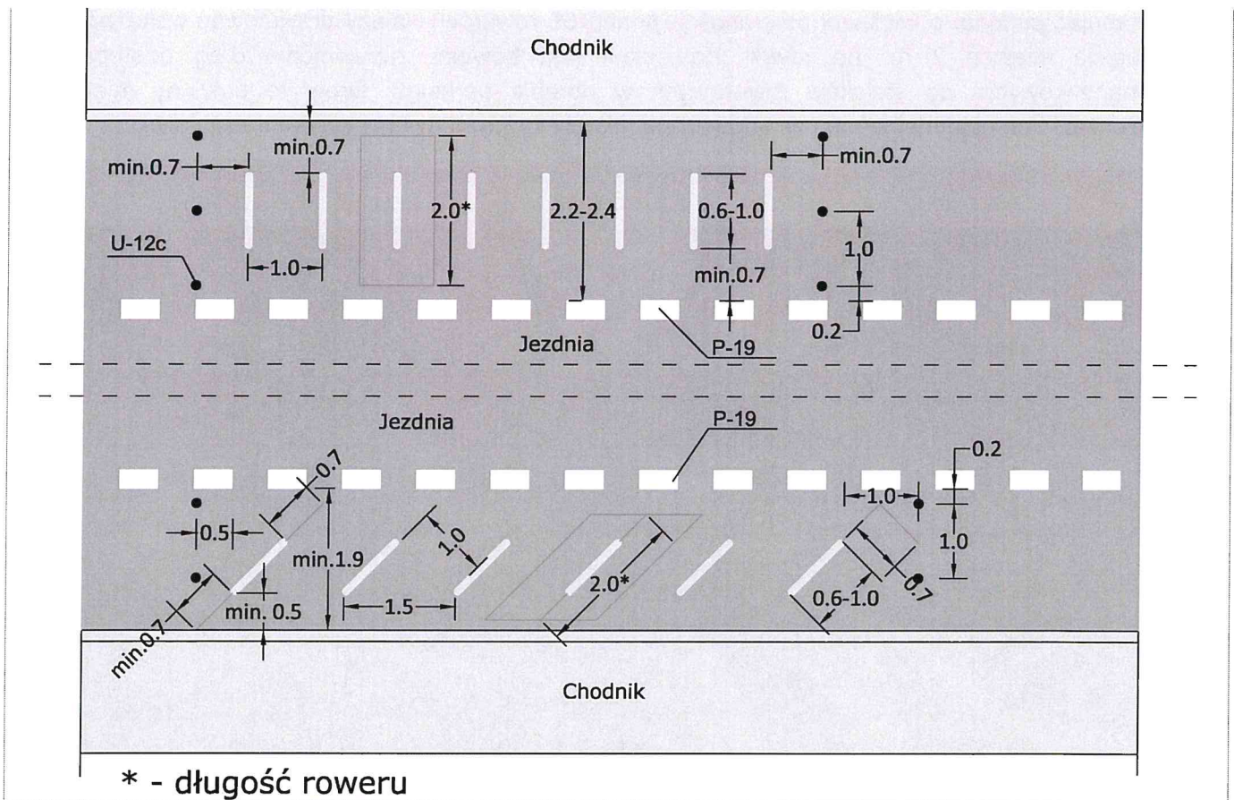
Rys. 25C. Sposoby organizacji parkingu rowerowego. Należy zachować minimalne odległości między stojakami oraz zapewnić wolną drogę dostępu (manewrową) umożliwiającą korzystanie z nich.
